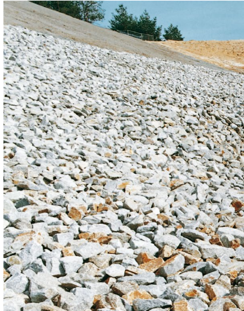
Auslaufbauwerk – Auslaufgerinne
